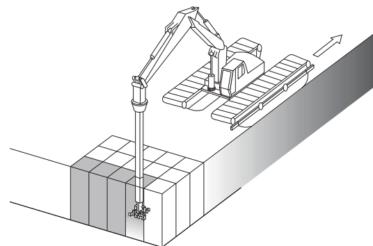
(VII) A R M 工法 自動ロータリー式施工法 ( \ell=4\text{m} , \ell=5\text{m} )
